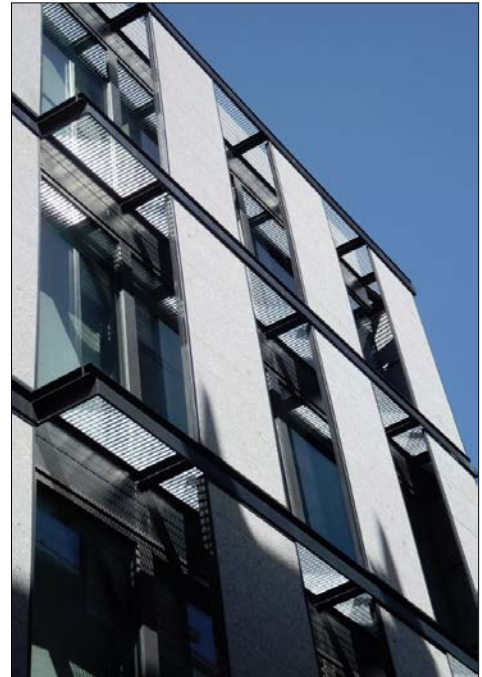
Fig.10: Fachada con vidrio termoacústico y paneles exteriores de granito sujetos a perfiles metálicos para dotar al edificio de sombreado
